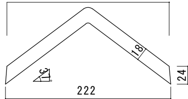
A-A 断面図
