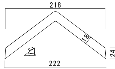
A-A 断面図
