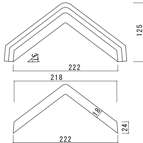
A-A 断面図
