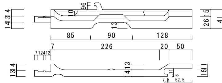
A-A 断面図
